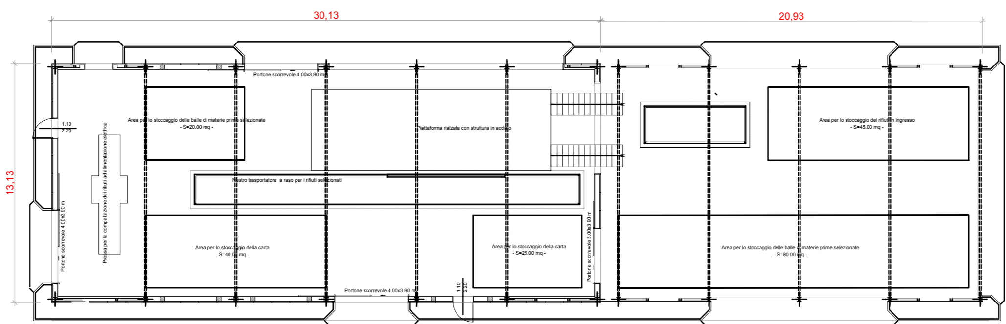
PIANTA INTERNA CAPANNONE IMPIANTO DI SELEZIONE E PRESSATURA
