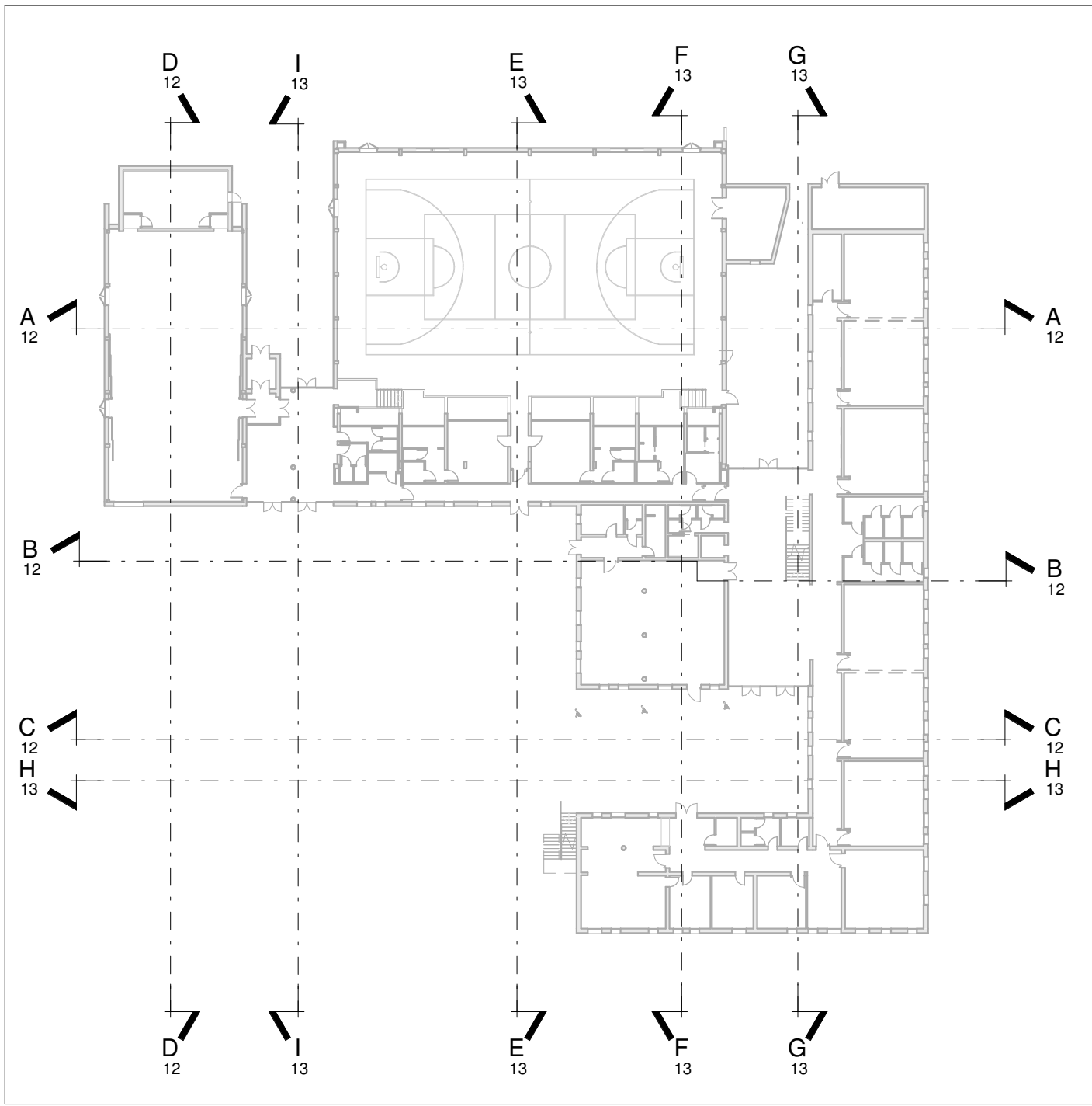
k-plan 1 : 500
