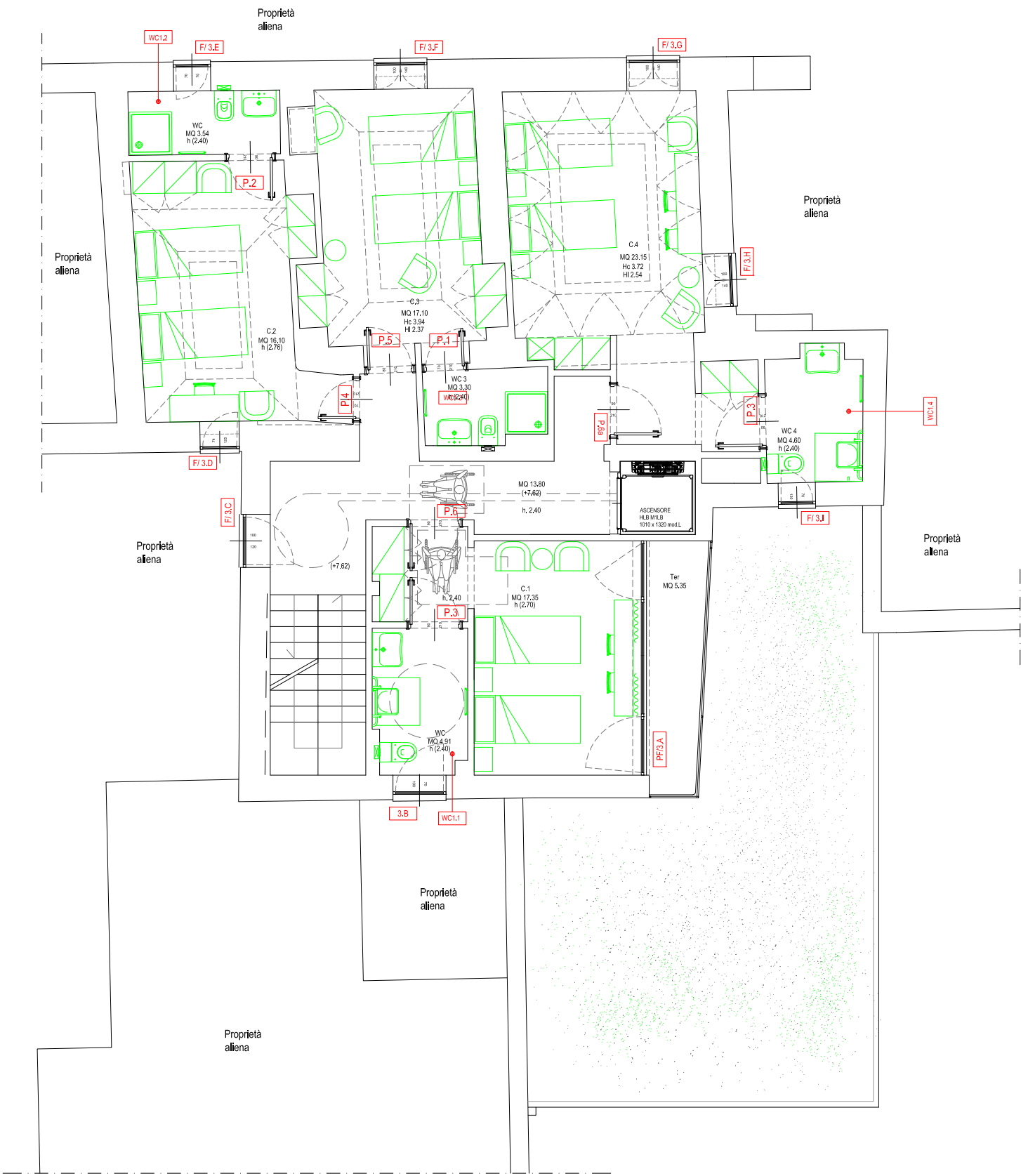
PIANO PRIMO PIANTA A QUOTA + 7.62
