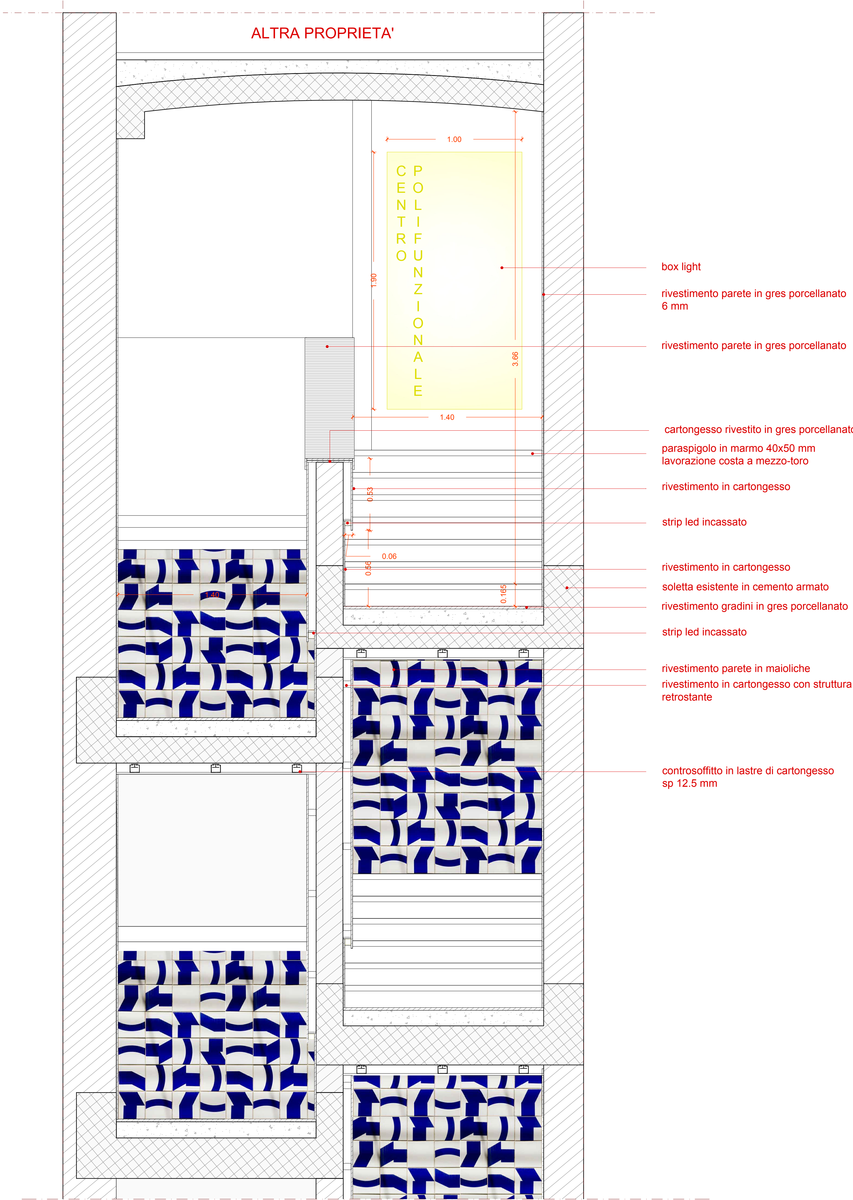
SEZIONE GG'_DETTAGLIO 1:10
