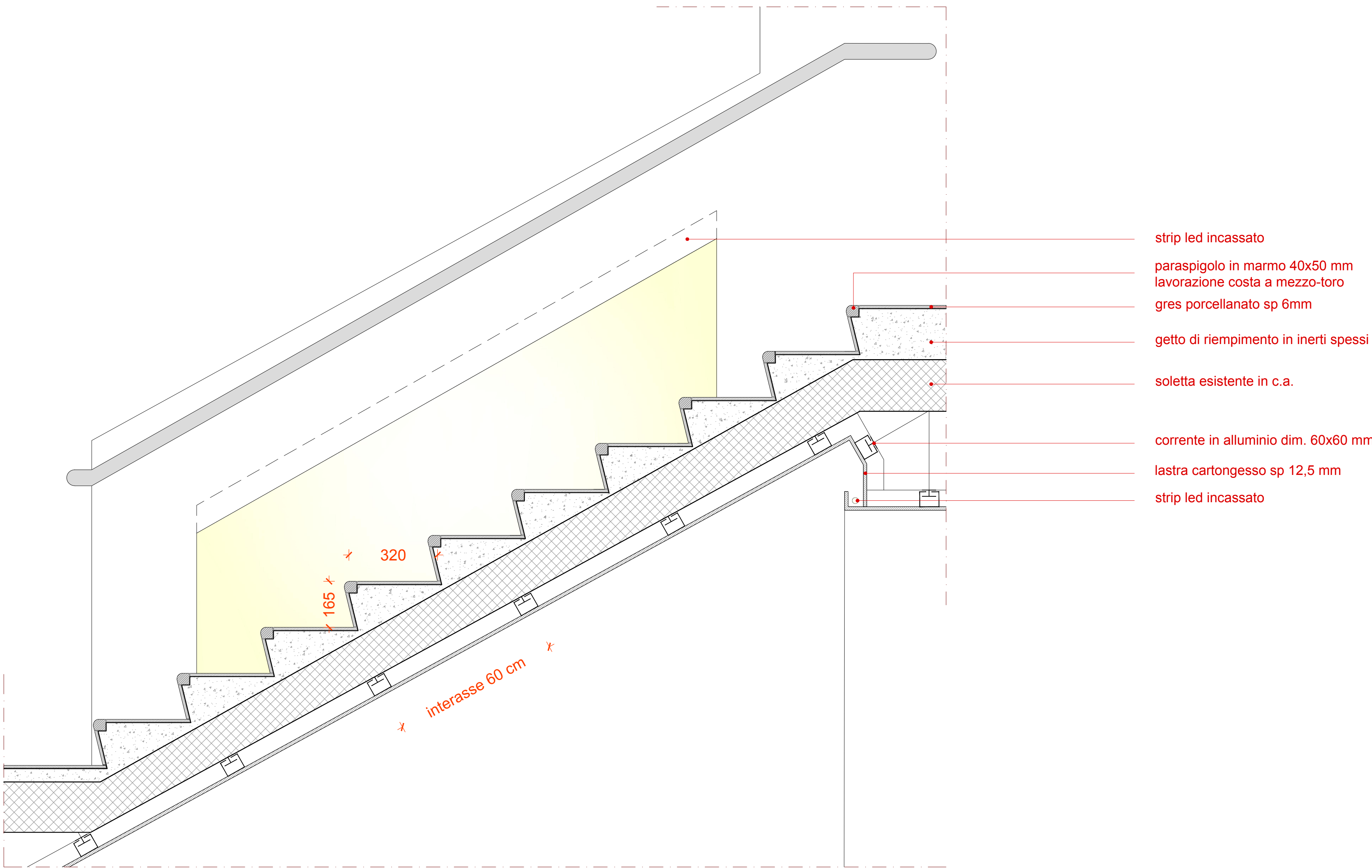
SEZIONE AA'_DETTAGLIO RAMPA 1:10
