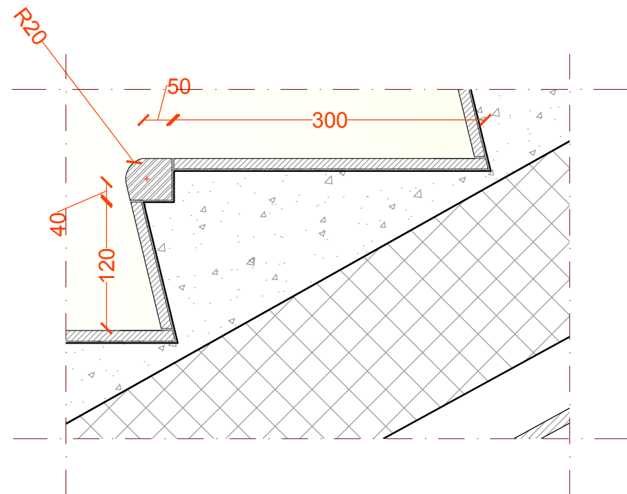
DETTAGLIO GRADINO TIPO 1:5
